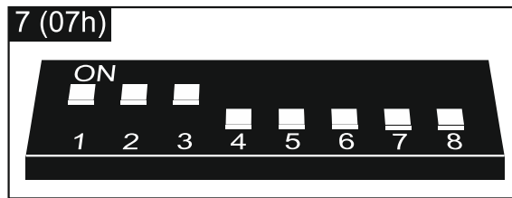
Rys. 5. Sposób ustawienia adresu w ekspanderze INT-RX-S / INT-RX.
